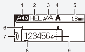
Displej LCD
